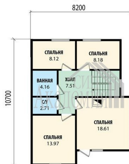
План второго этажа
