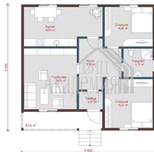
План 1-ого этажа
