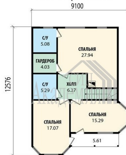
План второго этажа
