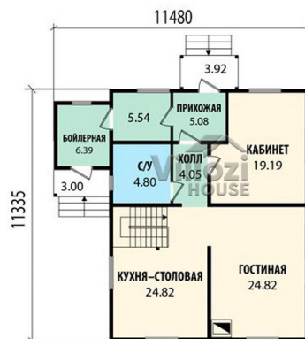
План первого этажа
