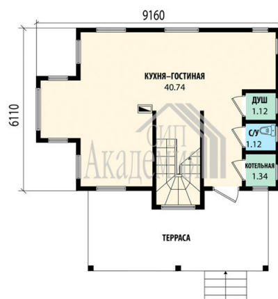
План первого этажа
