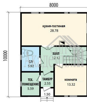
План первого этажа
