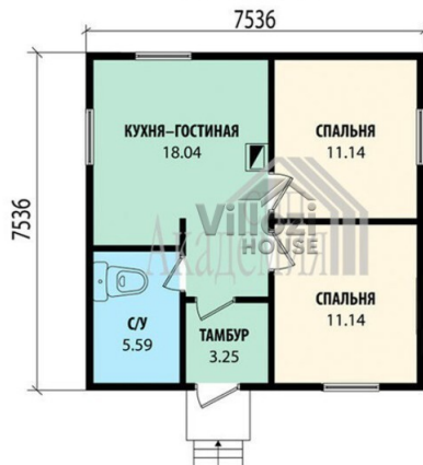
План первого этажа
