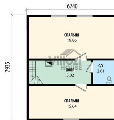
План второго этажа
