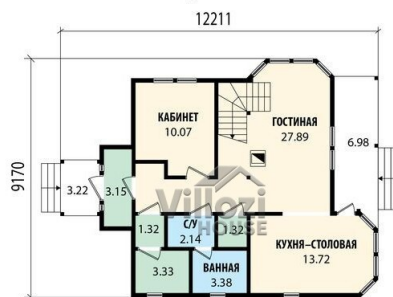
План первого этажа
