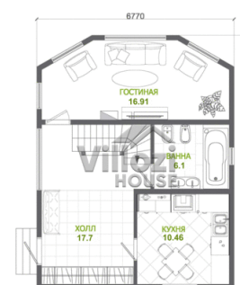
План 1 этажа
