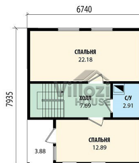
План второго этажа
