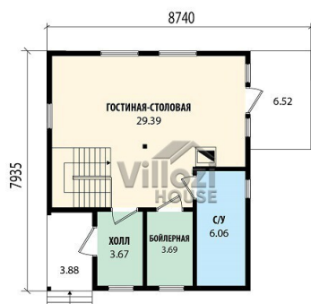
План первого этажа
