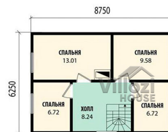
План второго этажа
