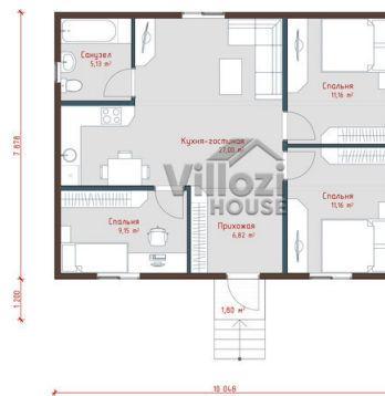
План 1-ого этажа
