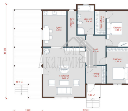
План 1-ого этажа
