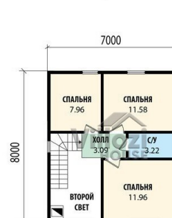
План второго этажа
