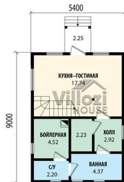
План первого этажа
