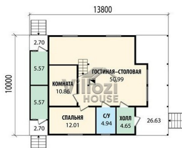
План первого этажа
