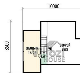
План второго этажа
