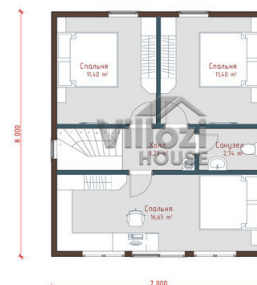
План 2-ого этажа
