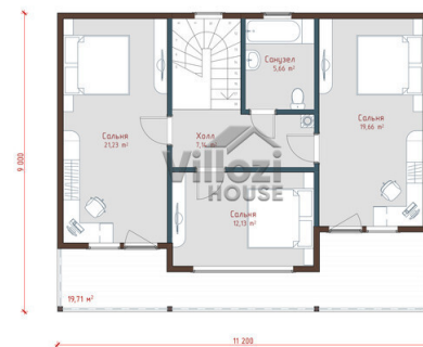
План 2-ого этажа
