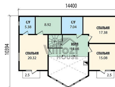
План второго этажа
