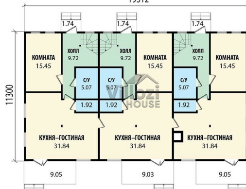
План 1 этажа 19512
