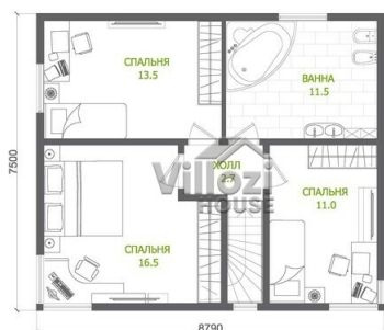
План 2 этажа
