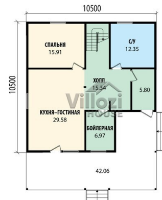
План первого этажа
