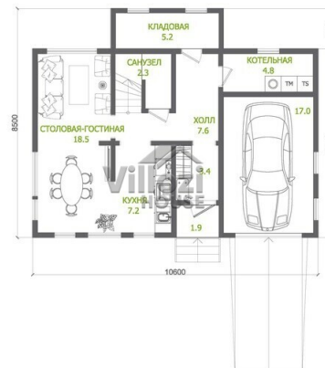
План 1 этажа
