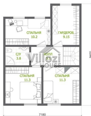
План 2 этажа
