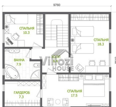
План 2 этажа
