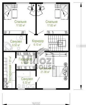
ПЛАН ВТОРОГО ЭТАЖА
